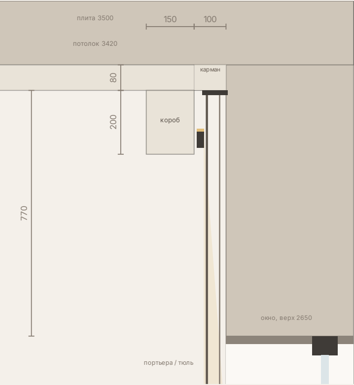
УЗЕЛ КАРНИЗА · РАЗРЕЗ ПО СЕВЕРНОЙ СТЕНЕ
